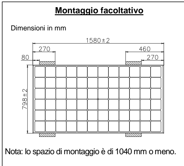
Figura 2-2: Montaggio facoltativo
