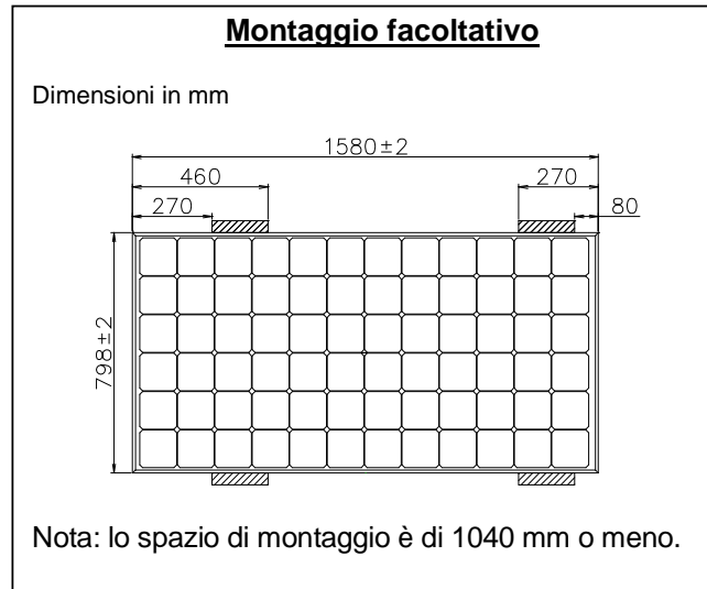
Figura 2-3: Montaggio facoltativo
