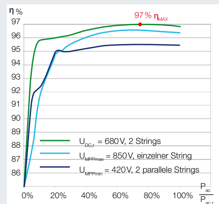
Wirkungsgradkennlinien PIKO 10.1
